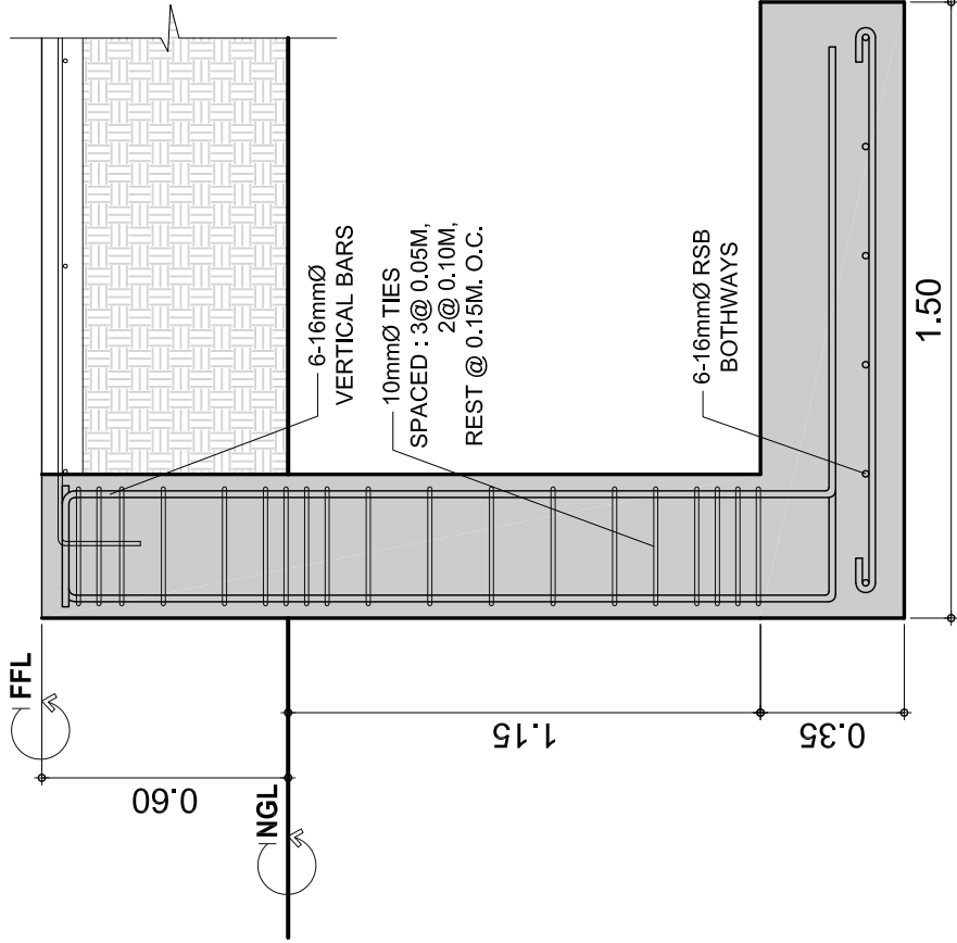
CF1 SECTION
